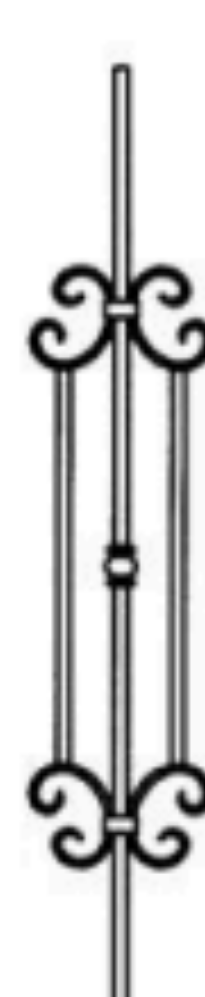
EIW 138 Ø14mm SCROLLS : 13 x 6mm 600 H x 200 W HEB / TBD / PL
