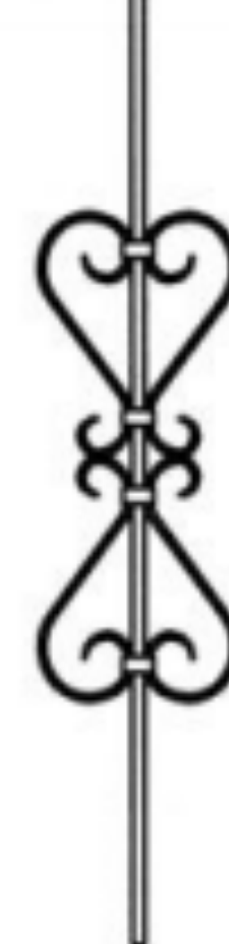
EIW 144 □12 / Ø14mm SCROLLS : 13 x 6mm 500 H x 202 W HEB / PL
